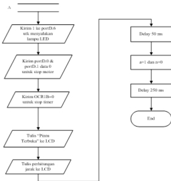
Gambar 8. Flowchart program tampilan pintu darurat terbuka
