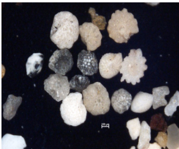
Gambar 4. Foraminifera bentik di titik lokasi BL16-001
