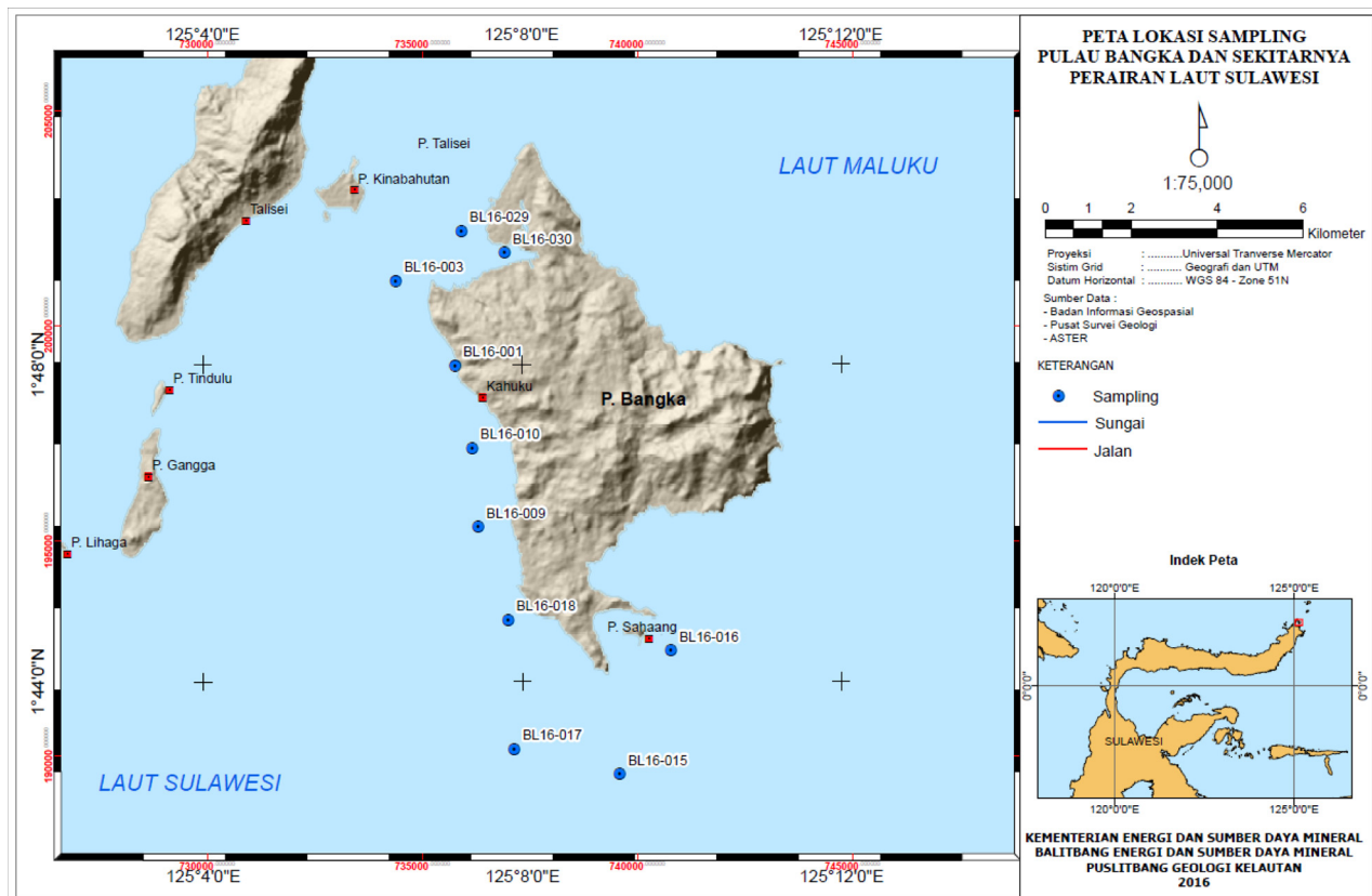
Gambar 1. Lokasi sampel sedimen untuk studi ostracoda
