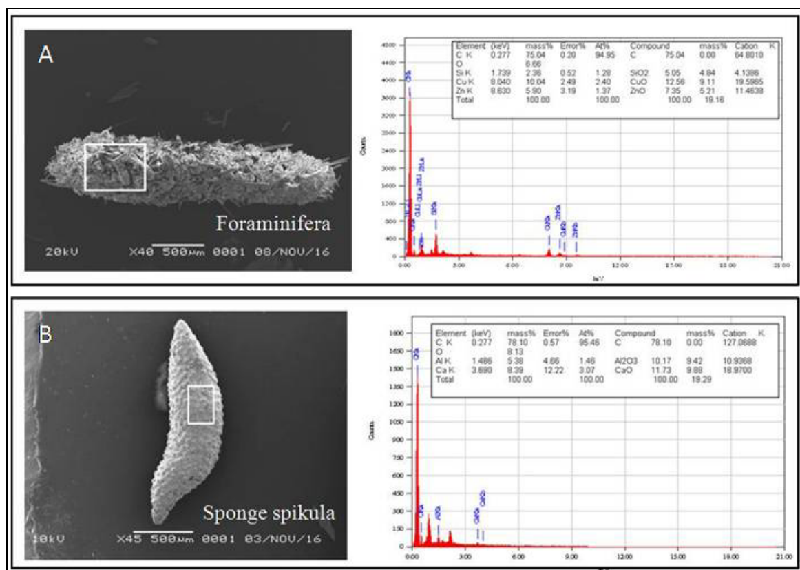
Gambar 5. Hasil uji SEM-EDX terhadap foraminifera dan sponge spikula
