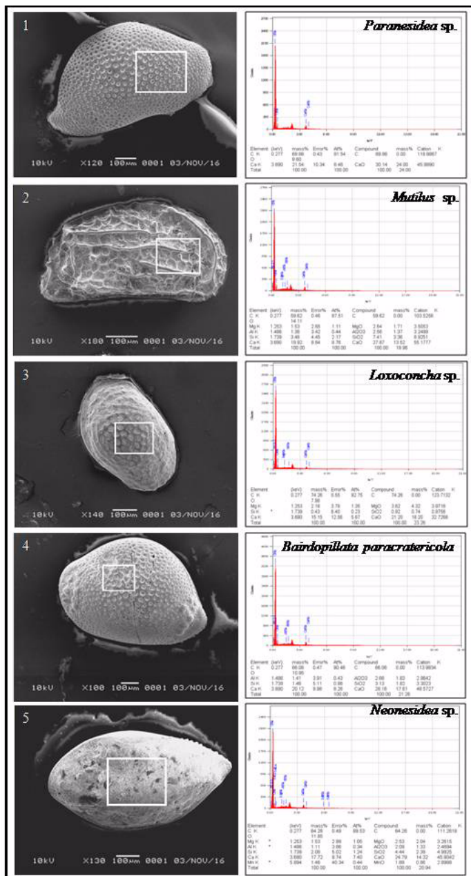
Gambar 3. Hasil uji SEM-EDX terhadap lima cangkang abnormal dari ostracoda
