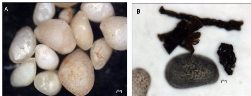
Gambar 2. Kondisi cangkang ostracoda di titik lokasi BL16-015 (A) dan BL16-30 (B)
