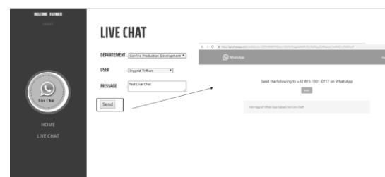
Gambar 7. Fitur livechat
