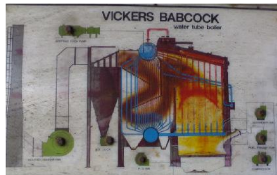
Gambar 1. Skema Ketel Pipa Air
