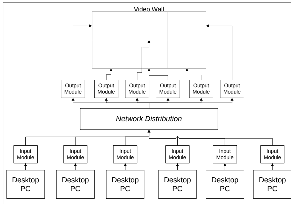
■ Gambar 3. Arsitektur Network Distribution
