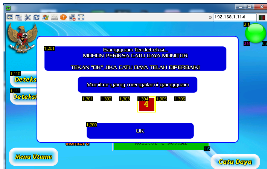
■ Gambar 13. Hasil Pengujian Subprogram Koreksi Format Tampilan – 2
