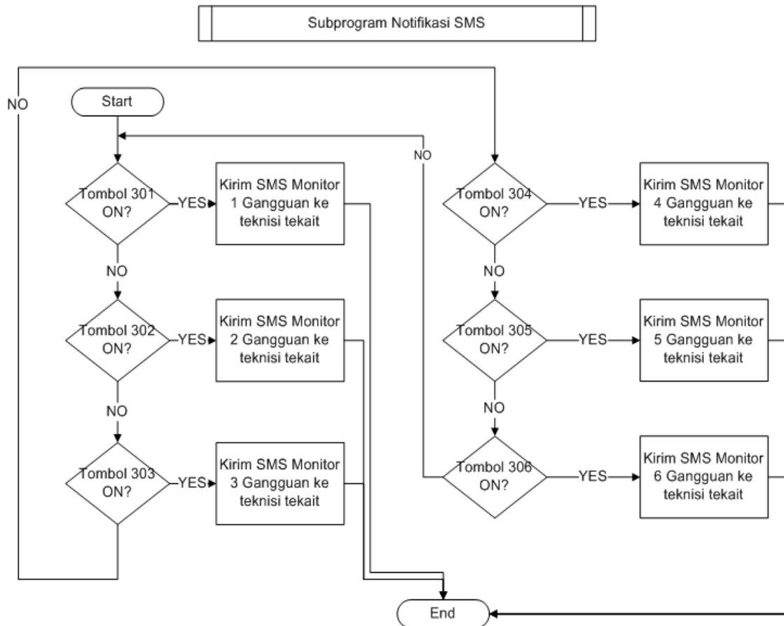
■ Gambar 8. Diagram Alir Subprogram Notifikasi SMS
