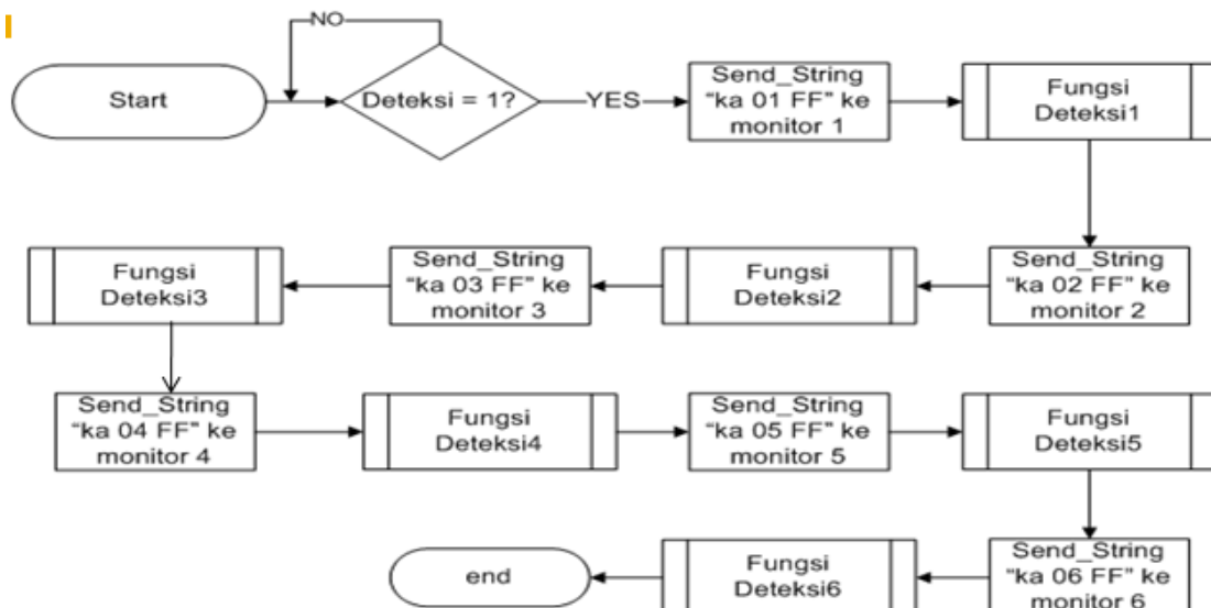
■ Gambar 6. Diagram Alir Subprogram Deteksi Gangguan
