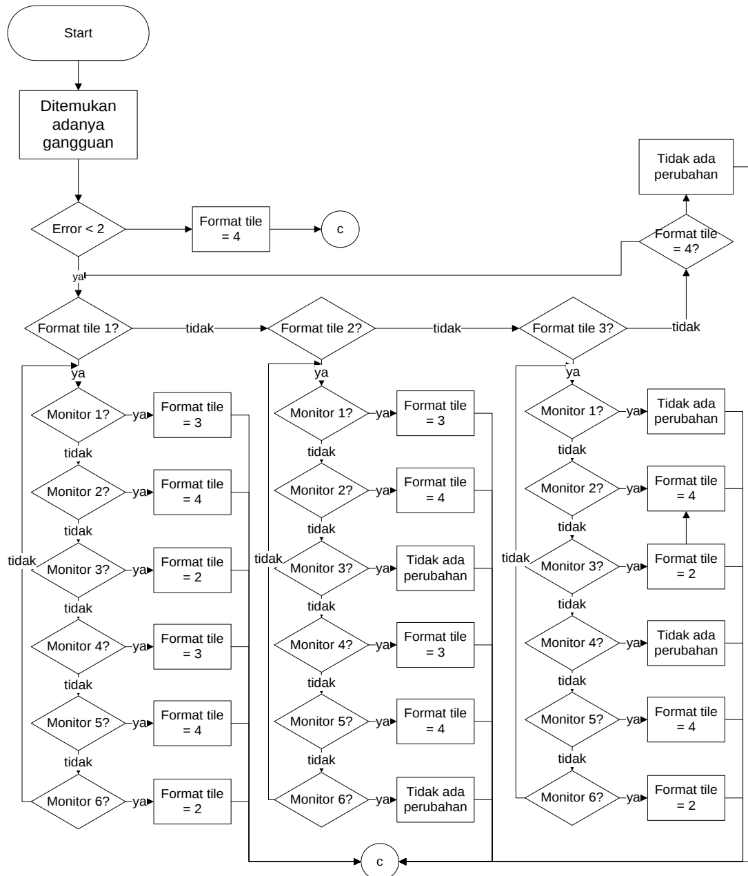
■ Gambar 7. Diagram Alir Perubahan Format Tampilan
