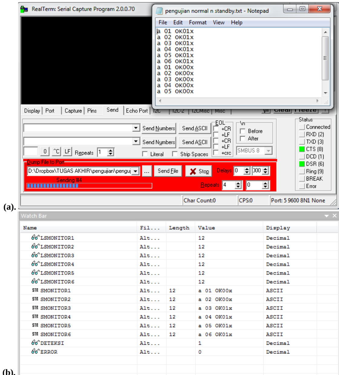
■ Gambar 10. (a) Hasil Pengujian Subprogram Deteksi – 2 (b) Hasil Pengujian Subprogram Deteksi – 3
