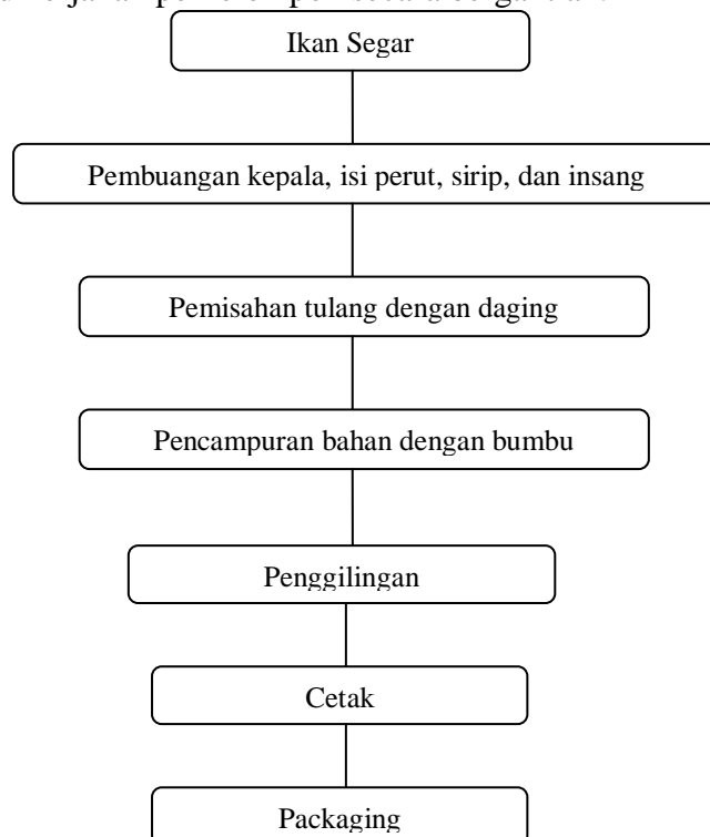
Gambar 1. Diagram Proses Pembuatan Nugget Ikan
