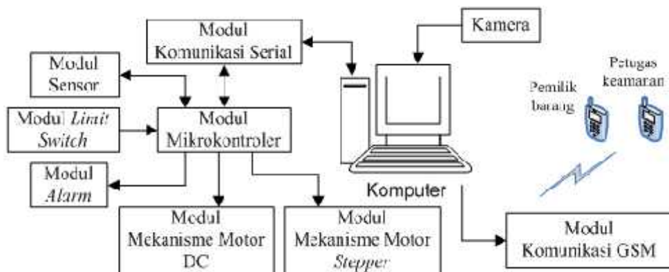
■ Gambar 4. Diagram Blok Rancangan
