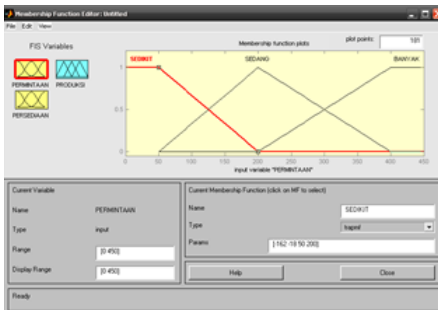
■ Gambar 9. Himpunan Variabel Fuzzy Permintaan Menggunakan Matlab
