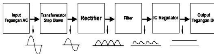
■ Gambar 6. Diagram Blok Catu Daya [4]
