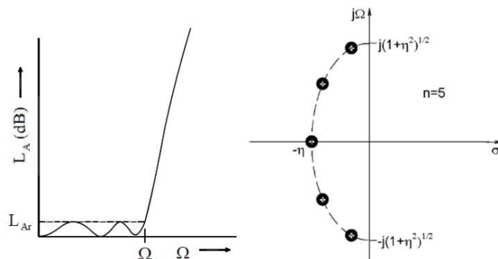
■ Gambar 4. Respon lowpass filter dan distribusi pole untuk pendekatan Chebyshev .
