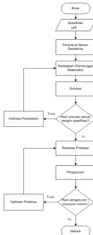
■ Gambar 6. Diagram Alir perancangan dan realisasi Lowpass stepped impedance .
