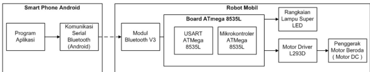
■ Gambar 1. Diagram Blok Pengendali Robot Beroda
