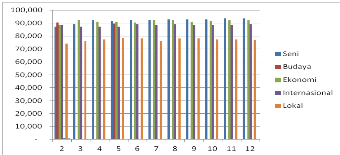
Gambar 7. Grafik Accuration pada c=5 dan k=11
