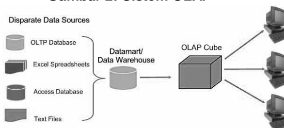
Gambar 2: Sistem OLAP
