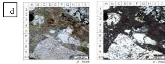
Gambar 5. Sayatan Petrografi pada(a) LP 81, (b) LP 14, (c) ST 14, dan (d) ST 70.
