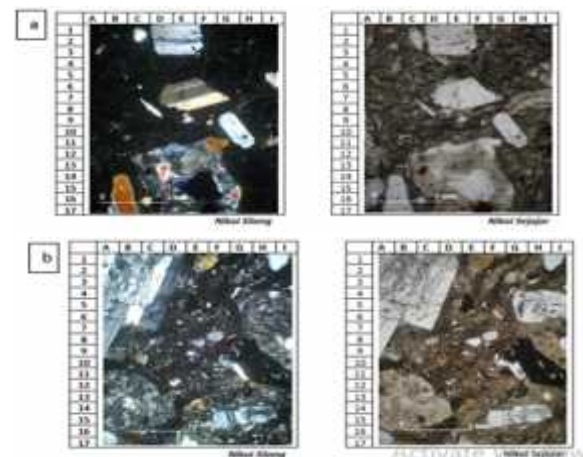
Gambar 6. SayatanPetrografi(a) LP 59, dan (b) LP 108.
