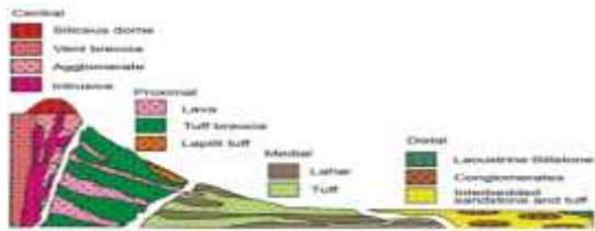
Gambar 2. Tipe-tipe fasies gunung api dan komposisi batuan penyusunnya [4].
