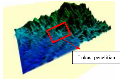
Gambar 3. Kenampakan 3D citra satelit SRTM daerah penelitian.
