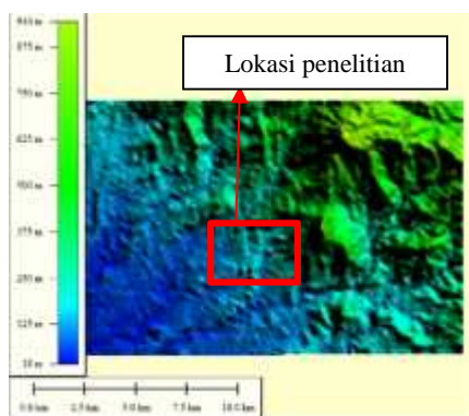
Gambar 4. Analisis Citra Satelit SRTM Lokasi Penelitian.
