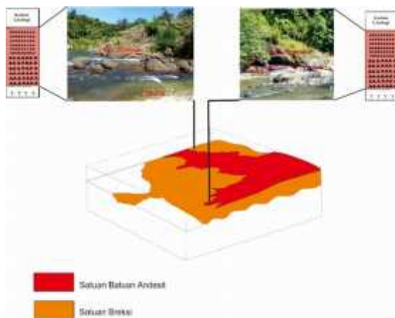
Gambar 7. Model Geologi dan Korelasi Stratigrafi daerah penelitian.
