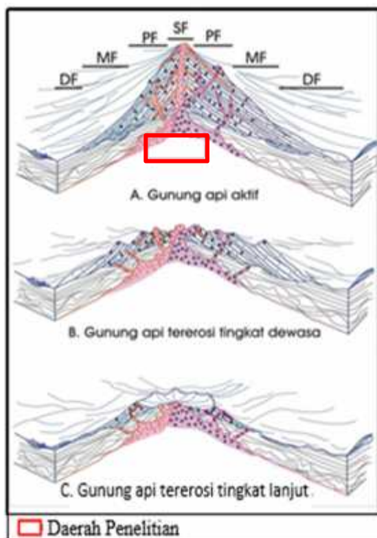
Gambar 8. Perkembangan bentang alam gunung api mulai dari bentuk gunung api aktif masa kini (A), Bentuk bentang alam gunung api telah tererosi pada tingkat dewasa dan (B), Bentang alam gunung api yang telah tererosi pada tingkat lanjut (C), Keterangan SF = Fasies Pusat; PF = Fasies Proksi; MF = Fasies Medial; DF = Fasies Distal [6].
