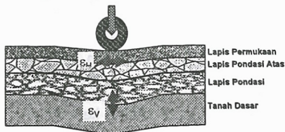
Gambar 1. Ilustrasi Respon Perkerasan Terhadap Beban Lalu-lintas
