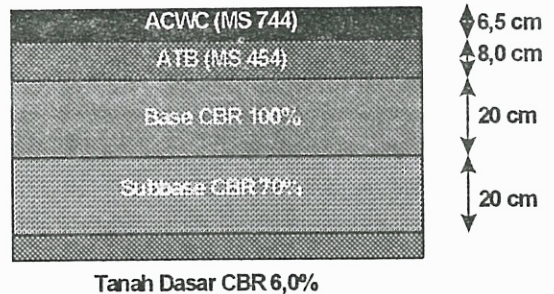
Gambar 2. Struktur perkerasan lentur untuk jalan baru berdasarkan hasil perencanaan
