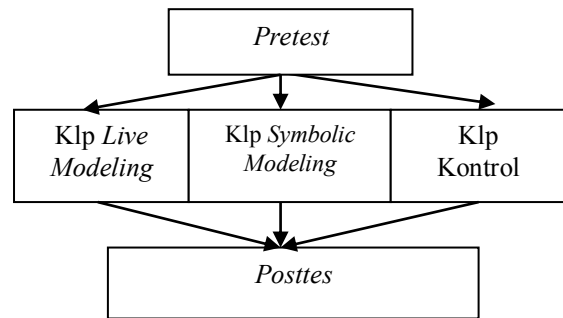
Gambar 1. Tahapan penelitian
