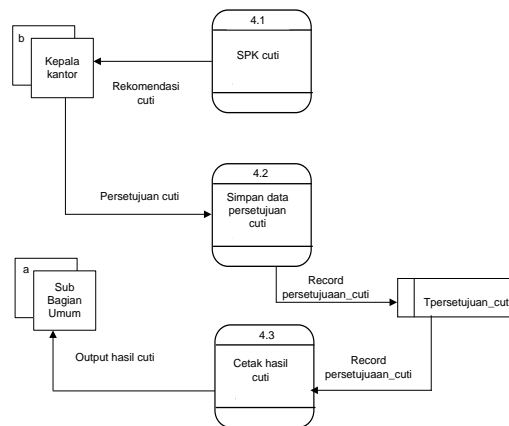
Gambar 3 DAD Level 2 proses persetujuan cuti
