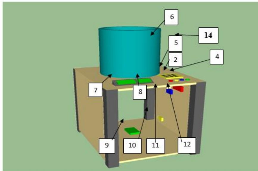
Gambar 3 Rancangan Bentuk Fisik Mesin penyaji beras secara digital
