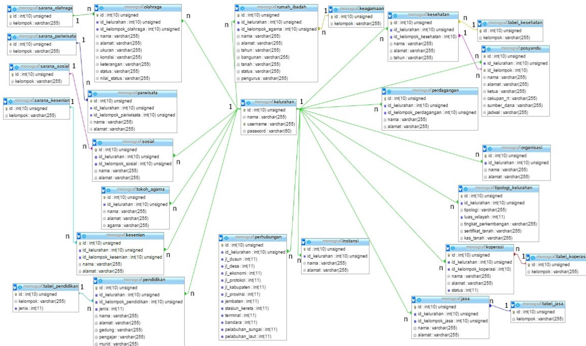
Gambar 4. Class Diagram monografi
