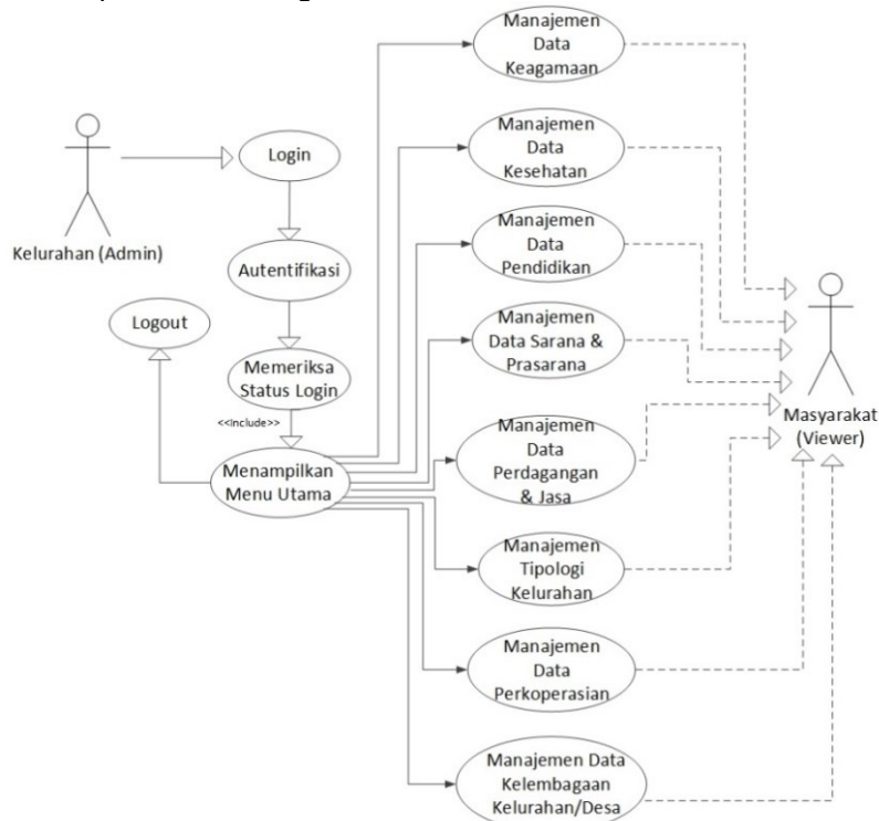
Gambar 2. Use-Case Monografi
