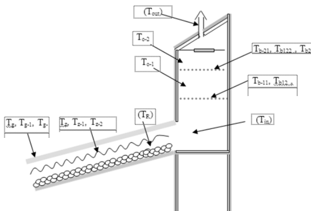
Gambar 1. Skema alat pengering yang digunakan.
