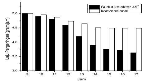
Gambar 2. Laju Pengeringan kolektor sudut 45° dibandingkan dengan pengeringan konvensional.
