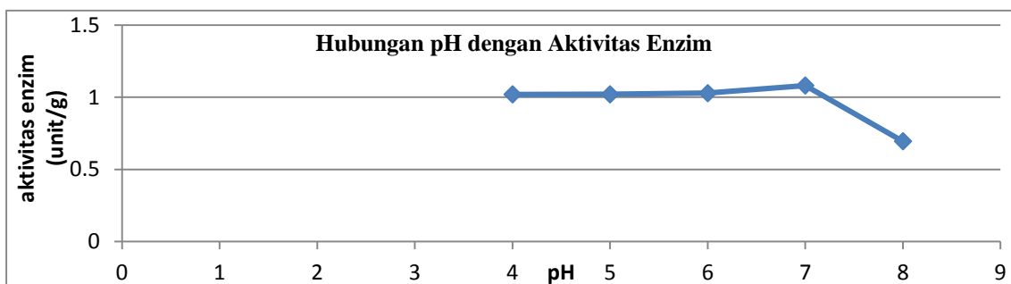
Gambar 2. Grafik Pengaruh pH terhadap Aktivitas Enzim Bromelin
