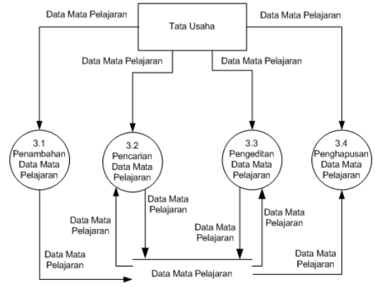
Gambar 4.5 DFD Level 1 Proses 3 Pengolahan Data Mata Pelajaran
