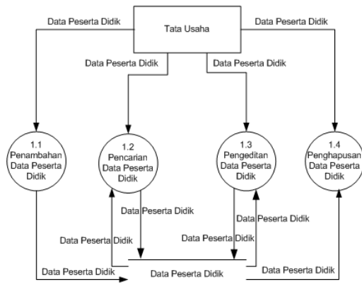
Gambar 4.3 DFD Level 1 Proses 1 Pengolahan Data Peserta didik
