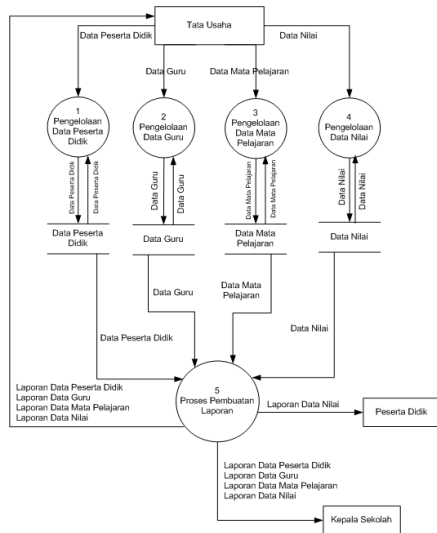
Gambar 4.2 DFD Level 1 Sistem Akademik Sekolah
