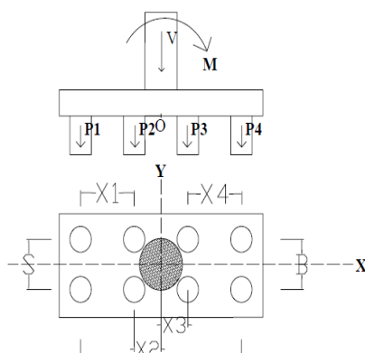
Gambar 2.15 Beban Vertikal dan Momen
