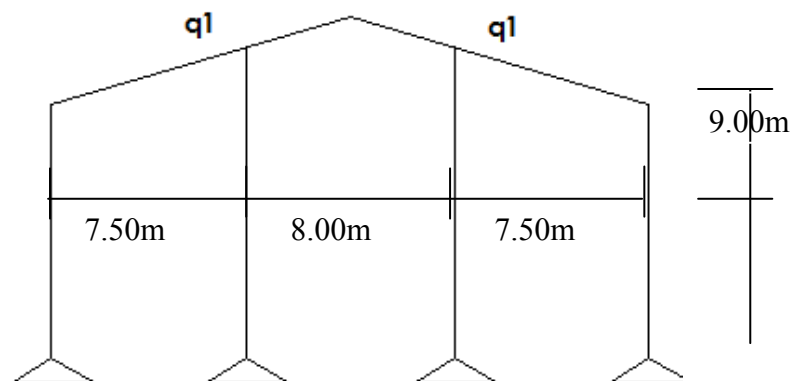
Gambar 4.4 Pembebanan Tetap
