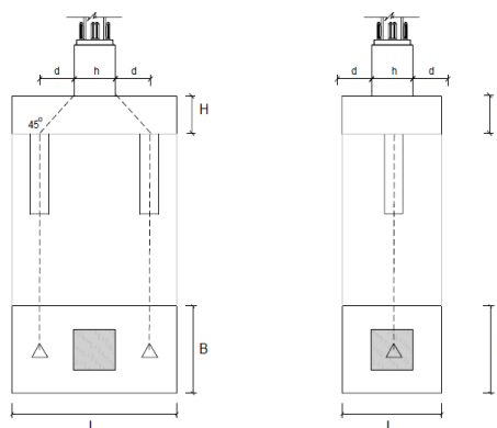
Gambar 2.16 Pile Cap
