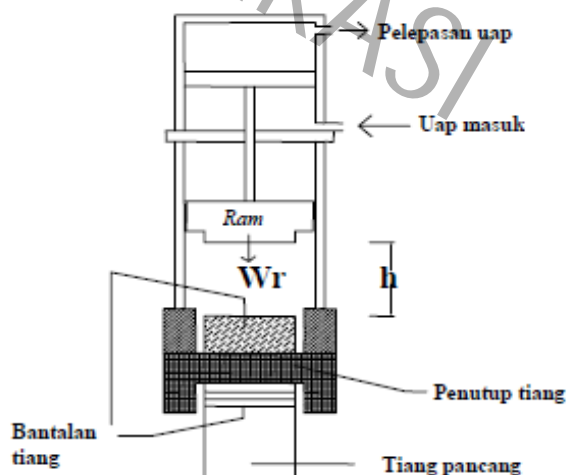
Gambar 4.6 Pemukul Tiang
