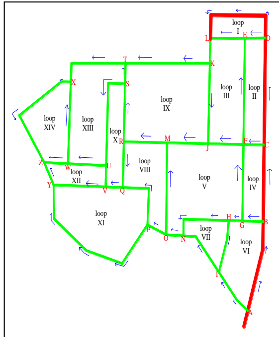
Gambar 2. Jaringan Air Bersih Pada Blok III (Loop)
