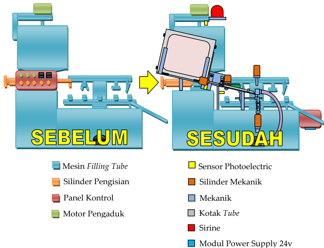
Gambar 8. Sketsa mesin filling tube sebelum dan sesudah dilakukan otomatisasi
