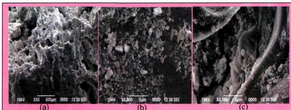
Foto 2. Scanning Electron Micrograph permukaan batu vulkanik pembesaran 5.000 x (a) batu vulkanik awal, (b) batu vulkanik diamobilisasi konsorsium bakteri anaerobik dan (c) batu vulkanik diamobilisasi konsorsium bakteri aerobik.
