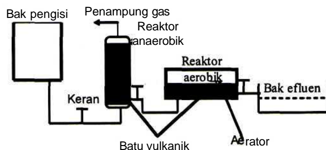
Gambar 1. Rancangan reaktor pengolahan limbah tekstil sistem kombinasi anaerobik-aerobik menggunakan biofilm konsorsium bakteri
