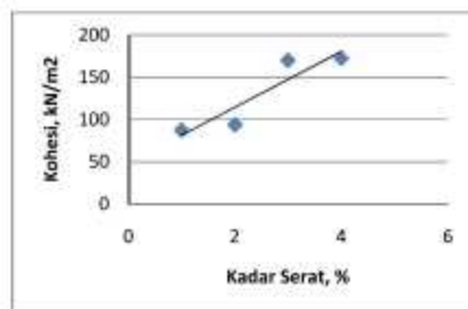
Gambar 3.4 Hubungan antara nilai kohesi terhadap kadar serat yang berbeda-beda.
