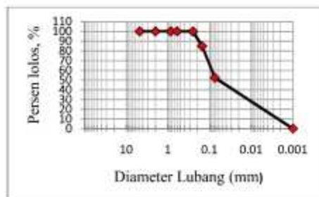
Gambar 3.1 Hubungan persentase lolos terhadap diameter lubang
