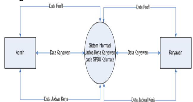
Gambar 4. Diagram Konteks
