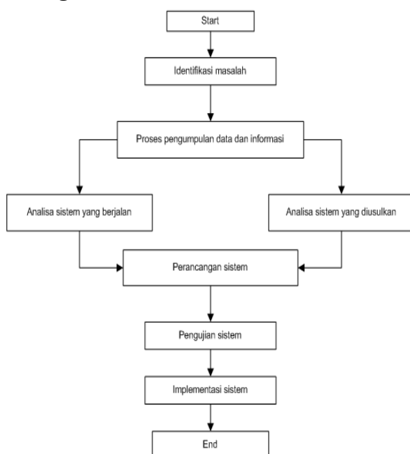
Gambar 1. Kerangka Penelitian
