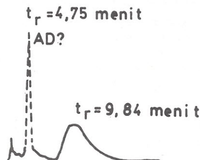
Gambar 7: Kromatogram Contoh Campuran Hasil Fermentasi Hari keenam ( H_6 ). Kondisi pemisahan sama dengan kondisi pada Gambar 4.
