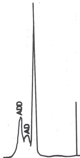
Gambar 1. Eluen: n-heksana-butanol-kloroform (5:3:1).
