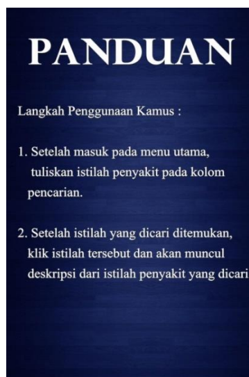
Gambar 18 Panduan
