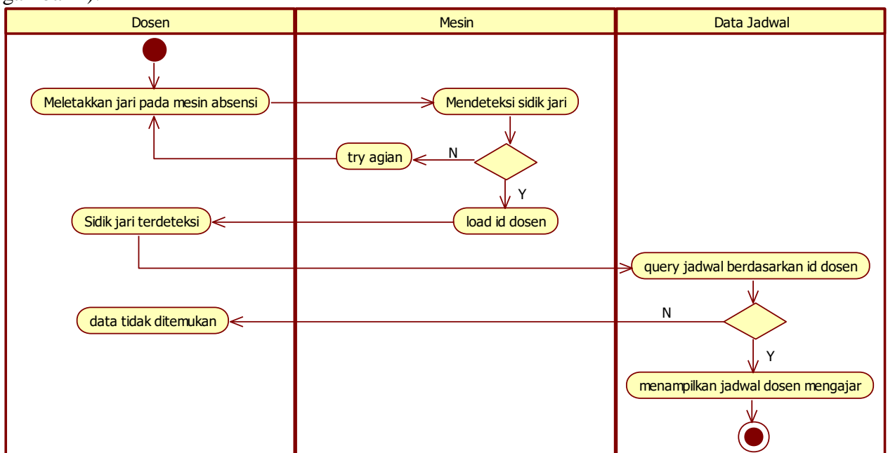
Gambar 4. Activity Diagram Integrasi Fingerprint System Dengan Real time Absensi
