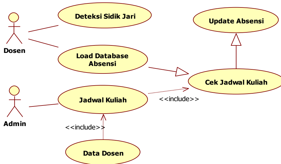
Gambar 3. Use case Diagram Integrasi Fingerprint System Dengan Real time Absensi
