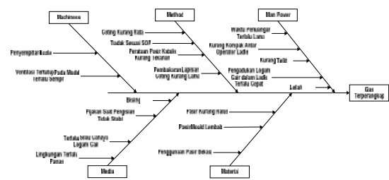
Gambar 9. FMEA Gas Terperangkap
