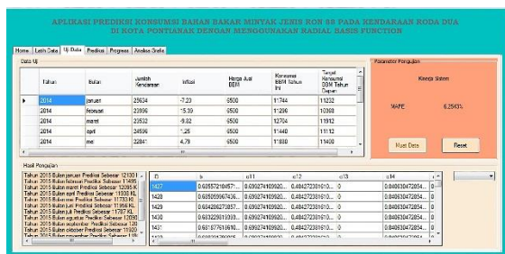
Gambar 5. Tampilan Pengujian Data
