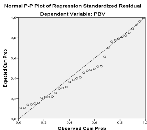
Gambar 4. Uji Normalitas
