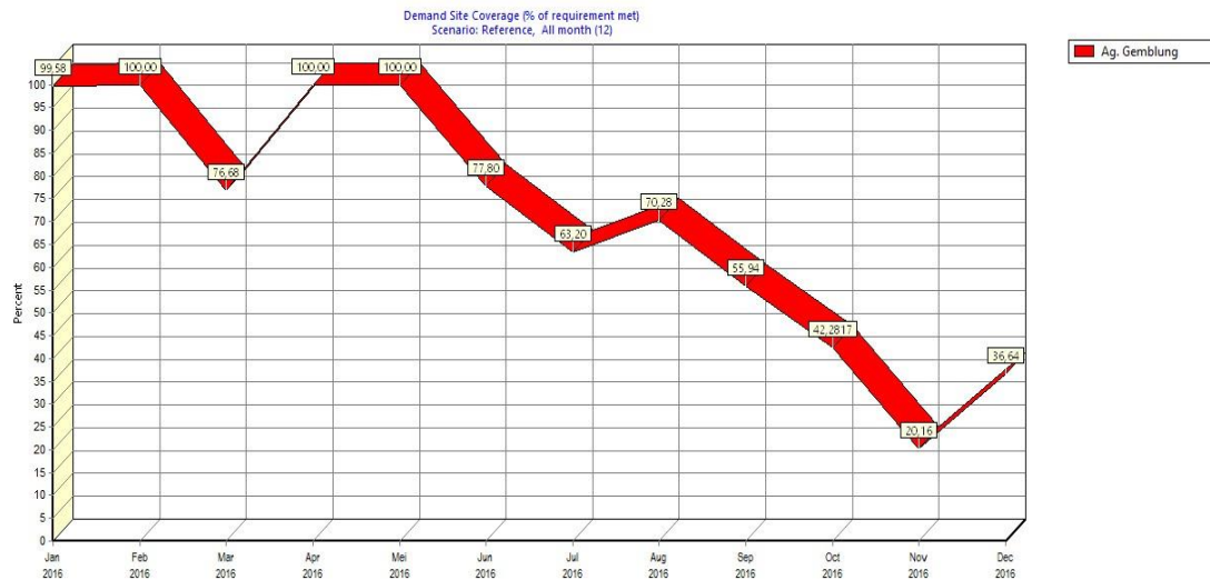
Gambar 6. Neraca Air Permukaan Bendung Gemblung dengan Water Evaluation and Planning
