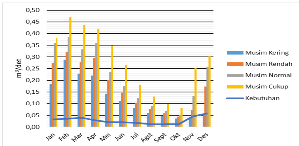
Gambar 5. Neraca Air Permukaan Bendung Gemblung dengan Microsoft Excel
