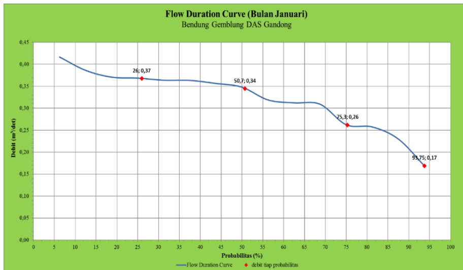
Gambar 4. Grafik Flow Duration Curve Bulan Januari Bendung Gemblung
