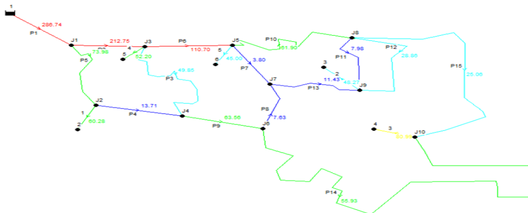
Gambar 7. Proyeksi perencanaan jaringan pipa distribusi Kota Sorong tahun 2026
