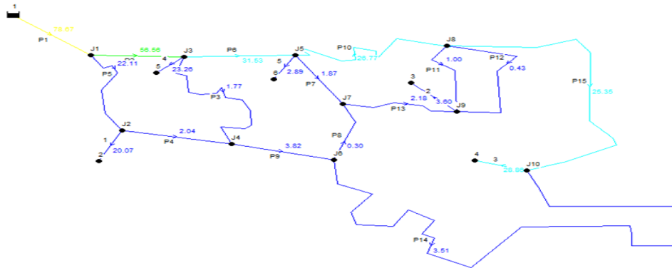
Gambar 6. Jaringan pipa Kota Sorong kondisi eksisting
