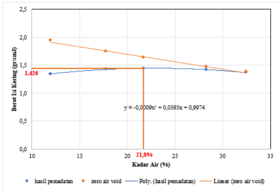
Gambar 5. Hasil Uji Pematatan
