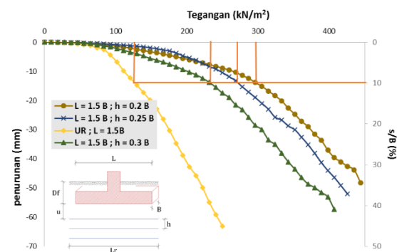
(b) L/B = 1,5
