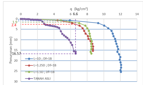
Gambar 11. Grafik Hubungan Tegangan dengan Penurunan Terhadap Kedalaman Kolom ( D_f ) = 15 cm
