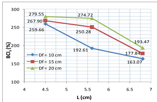
Gambar 8. Grafik Pengaruh Variasi Jarak antar Kolom terhadap Nilai BCI_s
