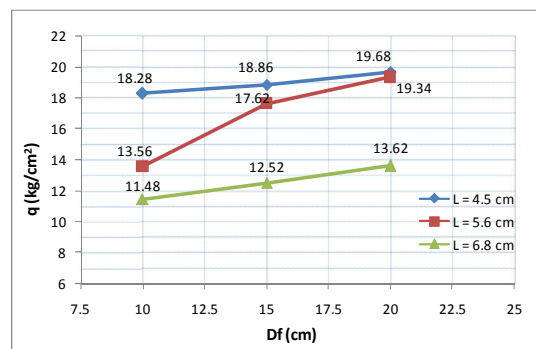
Gambar 5. Grafik Hubungan Tegangan Tanah pada Penurunan yang Sama terhadap Variasi Kedalaman Kolom
