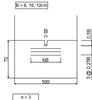
Gambar 2 pondasi dengan perkuatan
