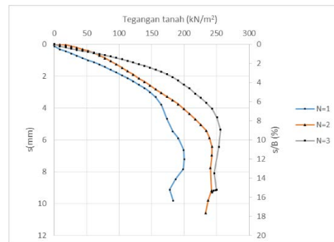
Gambar 6 Hubungan tegangan tanah dan penurunan dengan perkuatan pada lebar pondasi 6 cm
