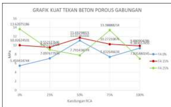
Gambar 7. Grafik kuat tekan beton porous.
