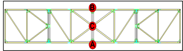
Gambar 3.1 Penamaan Titik Buhul pengukuran lendutan di tengah bentang
