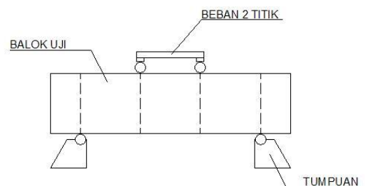
Gambar 3.2 Pembebanan 2 titik pada balok
