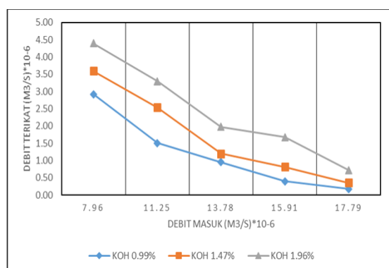
Gambar 4. Grafik hubungan debit masuk terhadap debit terikat \text{CO}_2 murni pada variasi konsentrasi KOH
