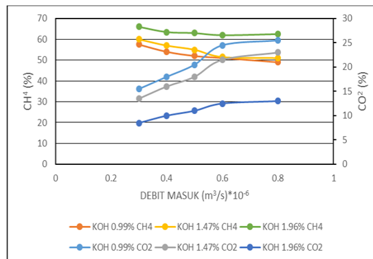
Gambar 8. Grafik hubungan debit masuk terhadap prosentase \text{CO}_2 dan \text{CH}_4 pada biogas dengan variasi konsentrasi KOH
