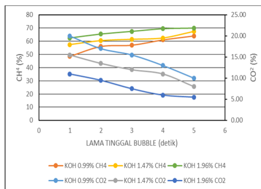
Gambar 6. Grafik hubungan lama tinggal bubble terhadap prosentase CO 2 dan CH 4 pada biogas dengan variasi konsentrasi KOH
