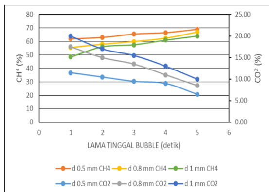
Gambar 7. Grafik hubungan lama tinggal bubble terhadap prosentase \text{CO}_2 dan \text{CH}_4 pada biogas dengan variasi lubang bubble generator
