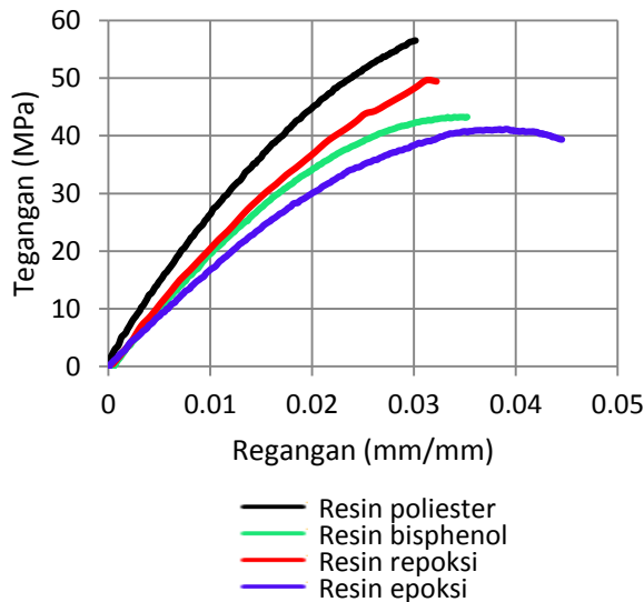
Gambar 5 Tegangan-regangan jenis resin tanpa serat
