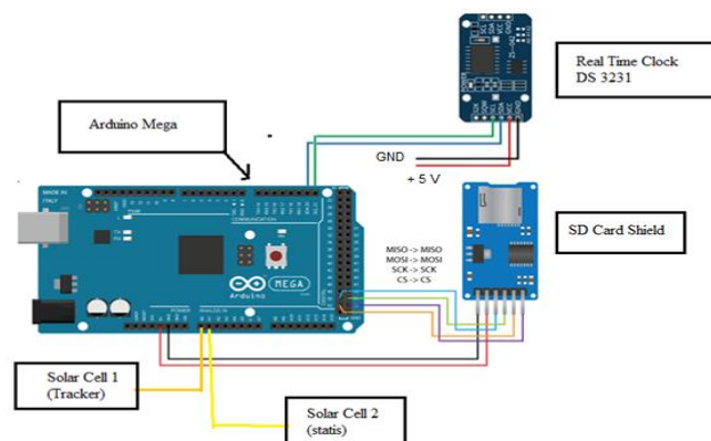
Gambar 7. Rangkaian akuisisi data dengan Arduino Mega, RTC DS 3231 dan SD Card
