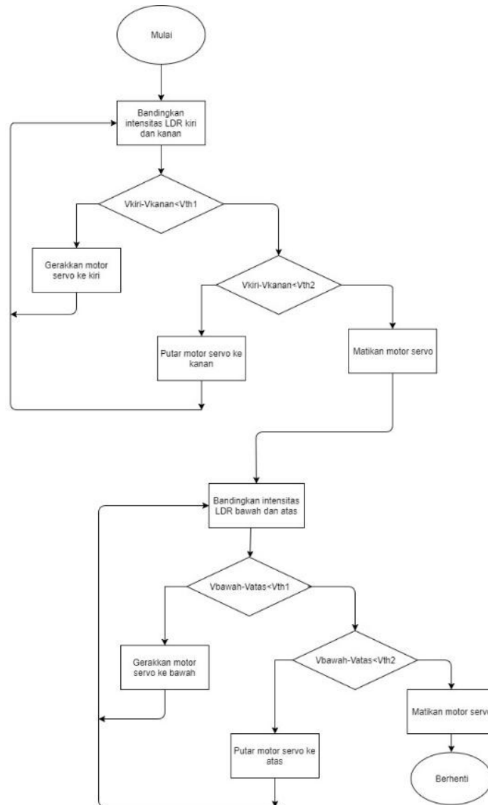
Gambar 6. Diagram alir pelacakan matahari dua sumbu
