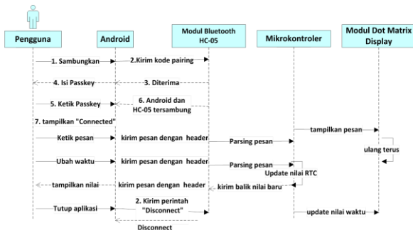
Gambar. 7 Sequence diagram aplikasi running text yang diusulkan
