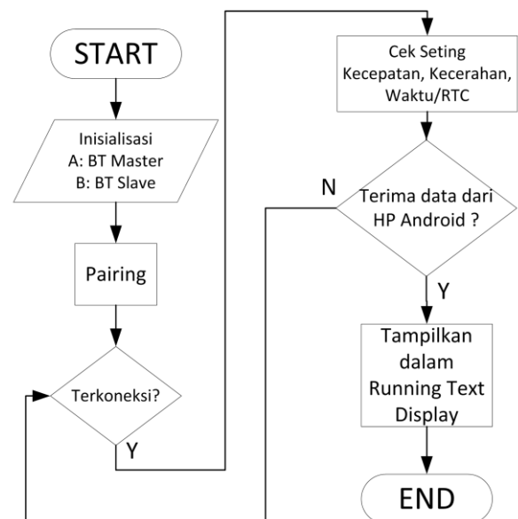
Gambar. 5 Diagram alir modul mikrokontroler dan bluetooth
