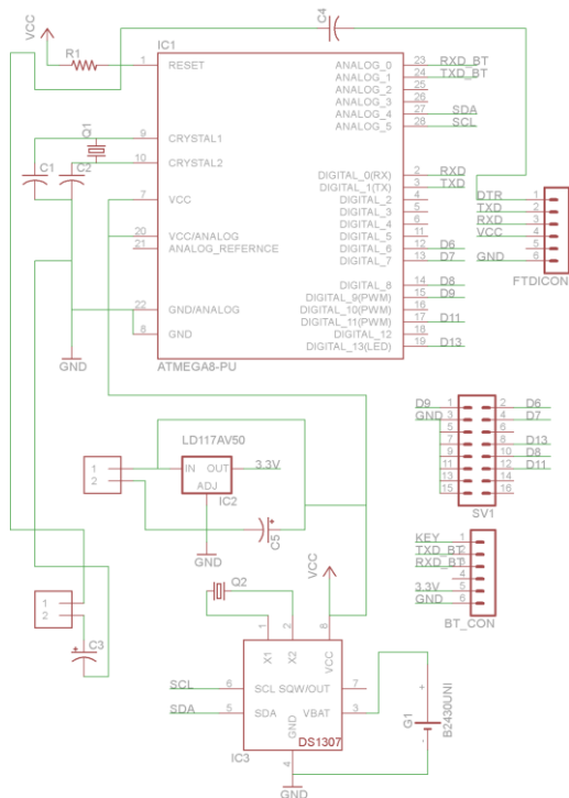
Gambar. 6 Skematik rangkaian kontroler
