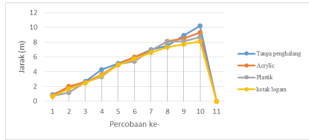
Gambar. 8 Data dikirimkan selama komunikasi dengan berbagai kondisi antara master dan slave
