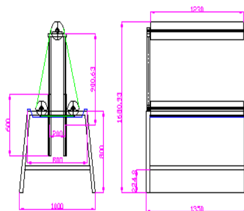
Gambar 10. Desain Mesin Pewarna Batik
