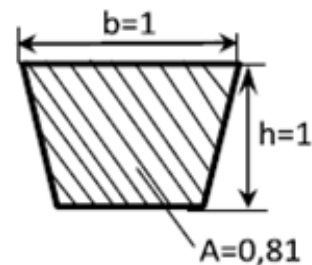
Gambar 3. Penampang Sabuk
