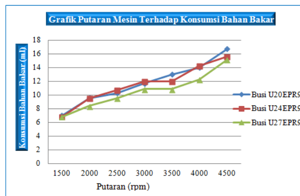
Gambar 2. Hubungan antara putaran mesin terhadap konsumsi bahan bakar
